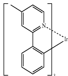
Ir(mppy) 3
