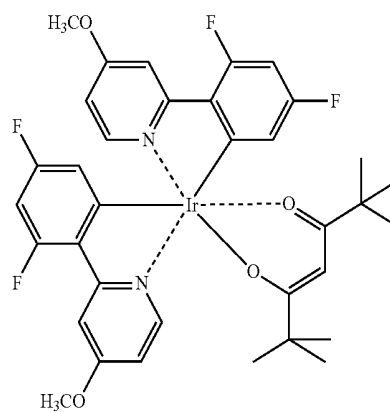
Ir(ppy) 3
