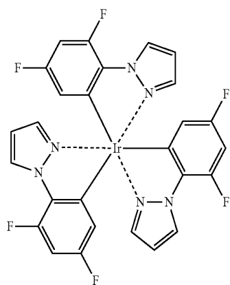
Ir(dfppz) 3
